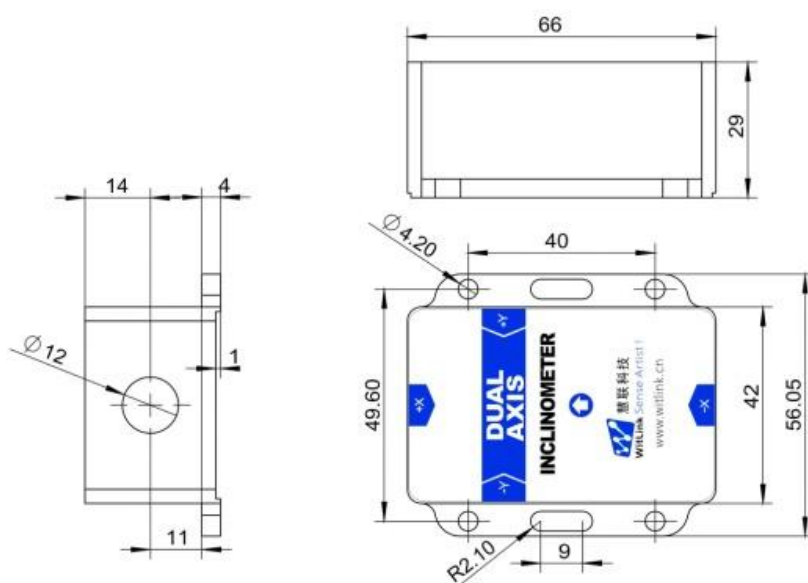
产品尺寸：L66mm×W56mm×H29mm
