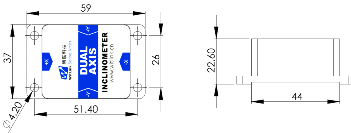
LIS326 产品尺寸 : L59 x W37 x H22.6 (mm)
